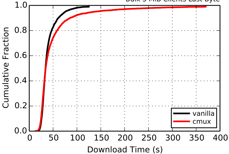
Bulk 5 MiB Clients Last Byte
