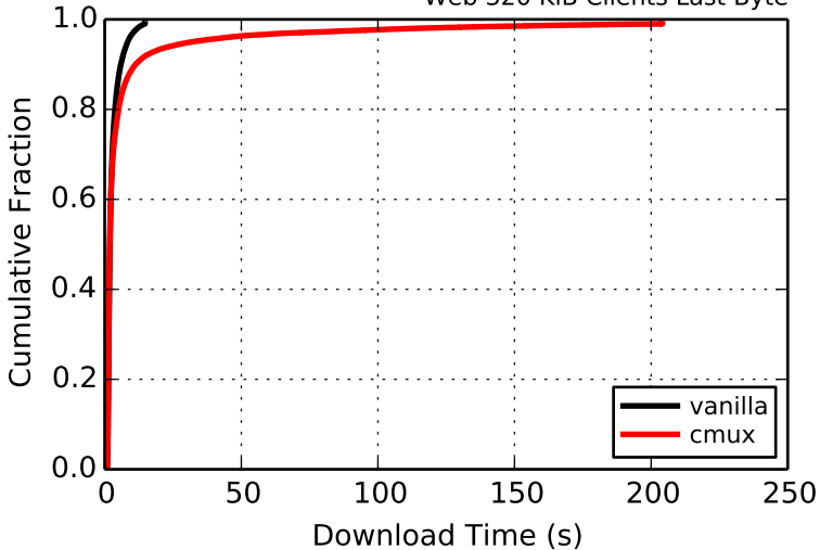
Web 320 KiB Clients Last Byte
