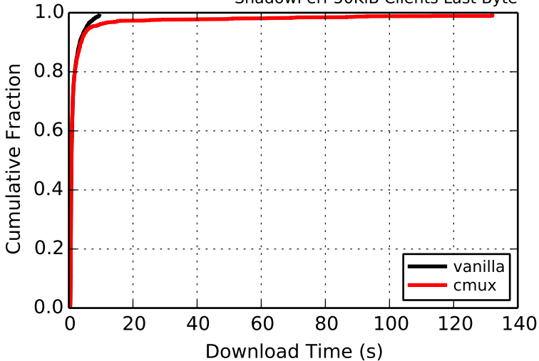
ShadowPerf 50KiB Clients Last Byte
